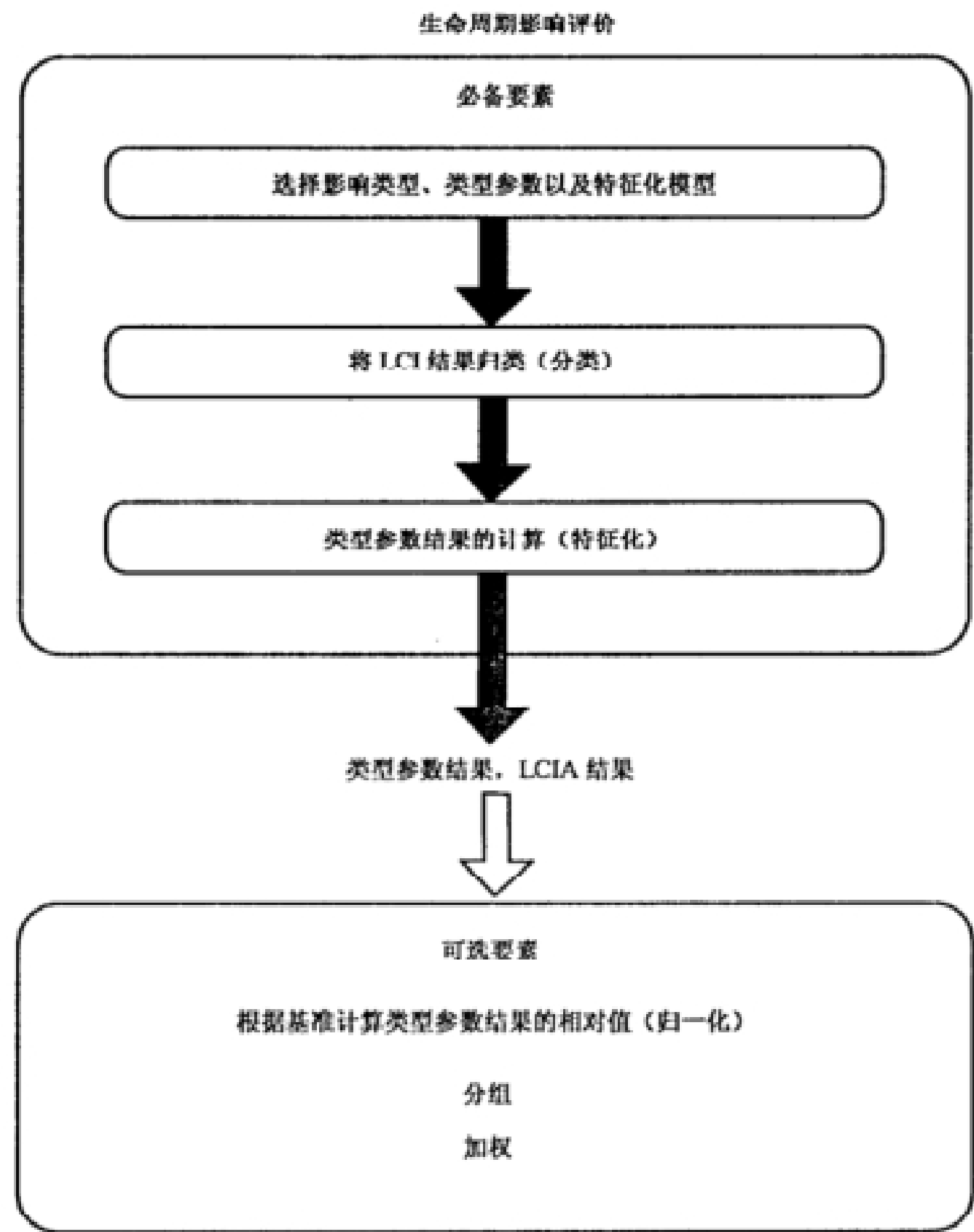
图 4 LCIA 阶段的要素
